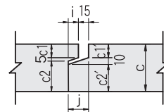
継手詳細図
